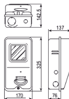
SAI CAJA EMPALME METALICA ENGANCHE DIN 7010-DRD
