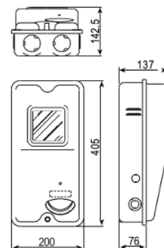
SAI CAJA EMPALME METALICA ENGANCHE AMERICANO 7010
